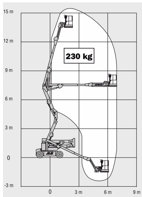
JLG E450AJ
