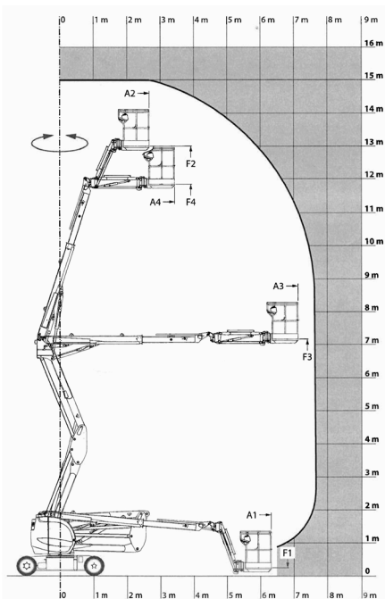
Manitou 150 ATEJC
